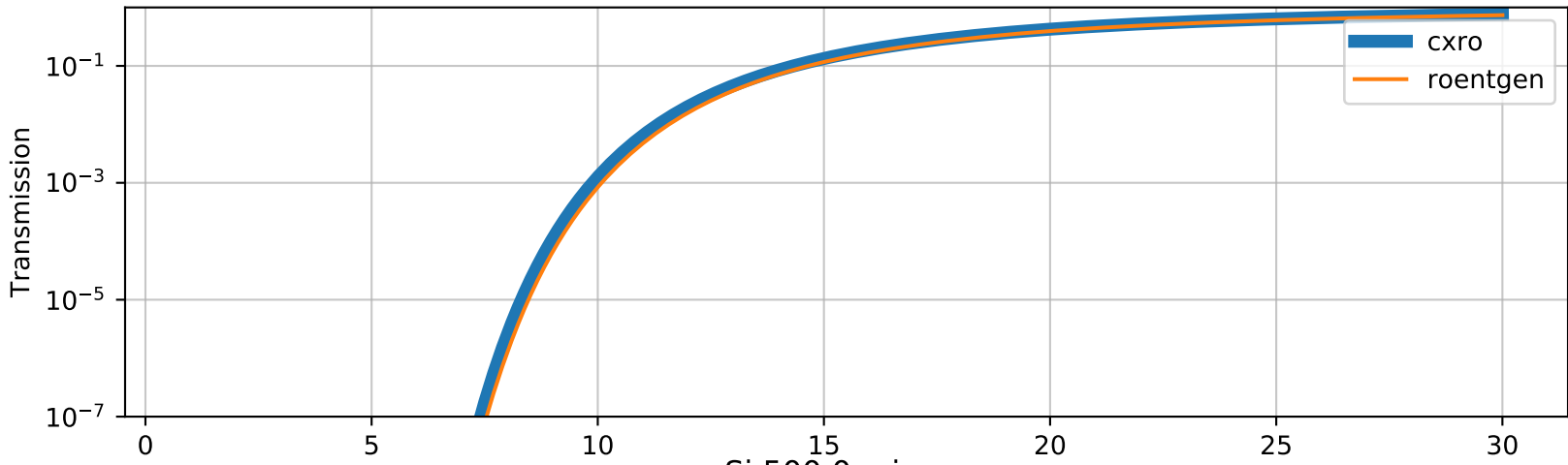
Si 500.0 micron
