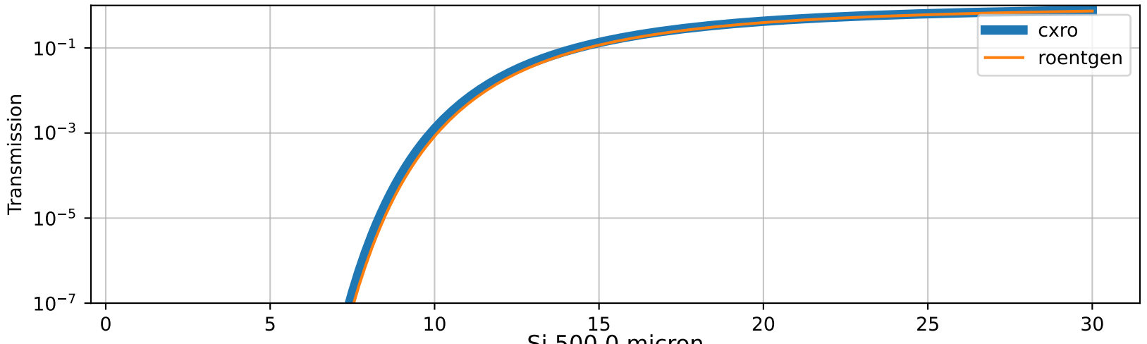
Si 500.0 micron
